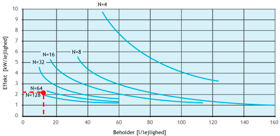
Figur 9. Dimensionering af varmtvandsbeholder med spiral til fjernvarme
